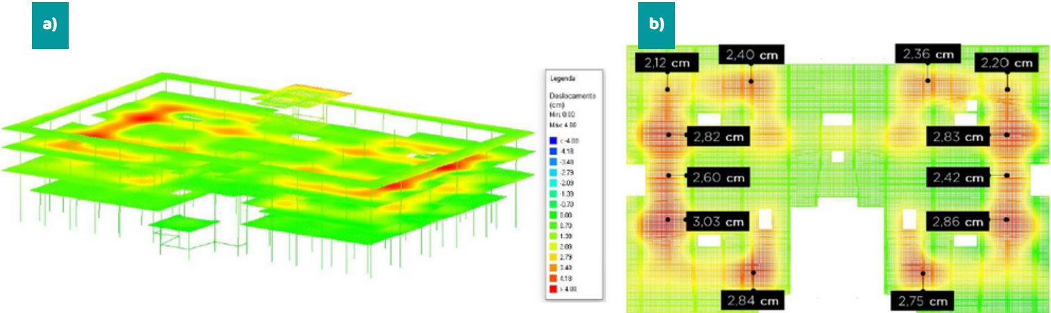
Fig.5- Análise computacional. a) Modelo analítico b) deslocamentos
