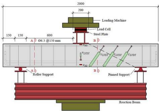
Fig.1- Sistema de ensaio
