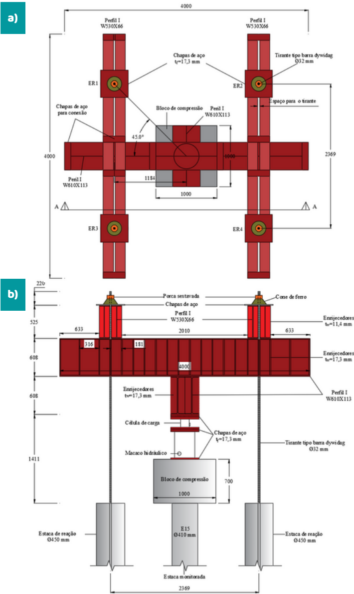
Fig.8- Sistema de reação. a) Planta baixa; b) Corte A-A.
