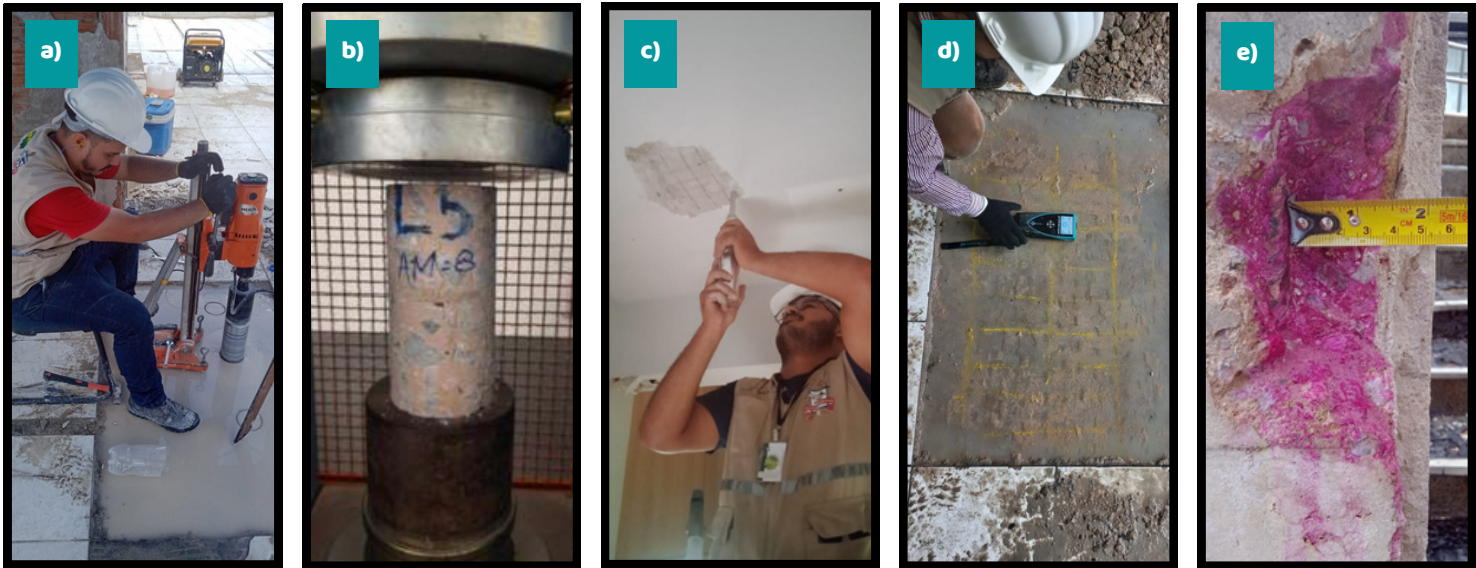
Fig.4- Ensaios a) Extração de testemunhos; b) Ensaios Testemunhos; c) Esclerometria; d) Pacometria; e) Carbonatação.
