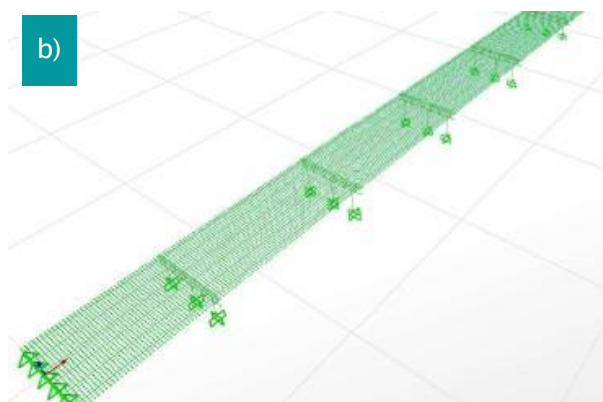
Fig.7- a) Ponte com estrutura mista b) Modelo analítico
