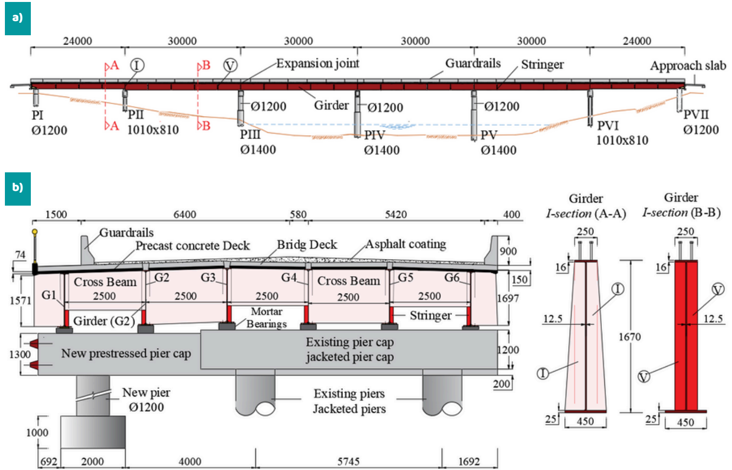
Fig.9- a) Perfil longitudinal; b) Seção transversal;
