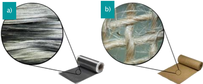
Fig.3- Reforço a) Manta de carbono; b) Tecido de juta.
